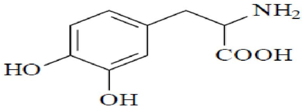
L-DOPA
